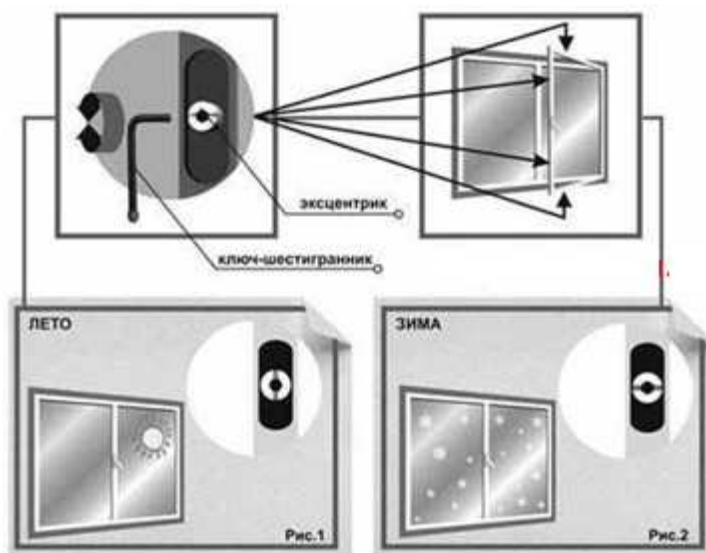
Рисунок 1. Переход пластикового окна из летнего режима в зимний и на оборот.
